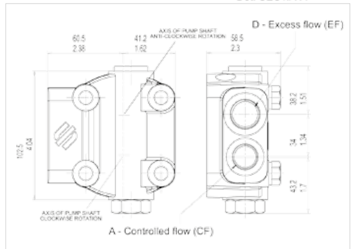
Det. SECTA-A
